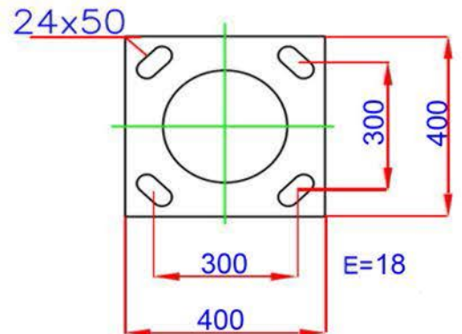
DETALLE PLACA BASE
