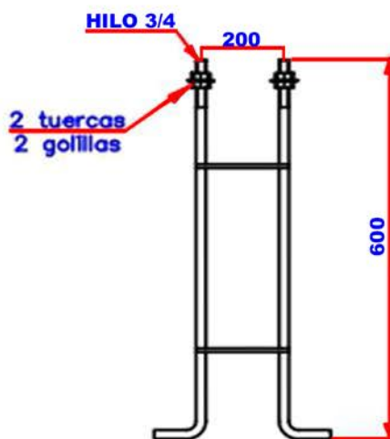
DETALLE CANASTILLO
